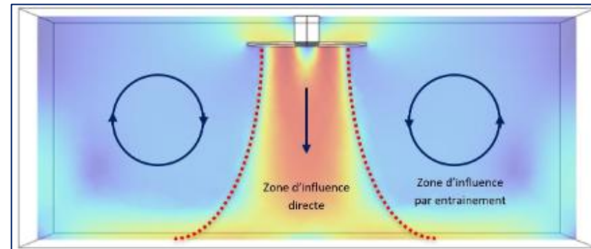
Schéma de l'écoulement d'air induit par un brasseur d'air soufflant vers le bas
